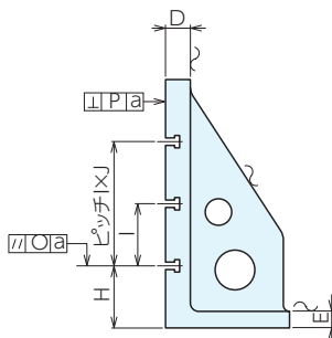
T溝詳細図
