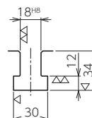
T溝詳細図
